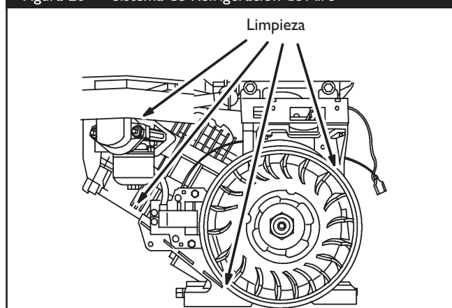
Figura 26 — Sistema de Refrigeración de Aire
